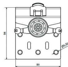
Top roller
