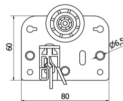
Bottom roller
