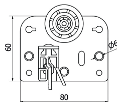
Bottom roller
