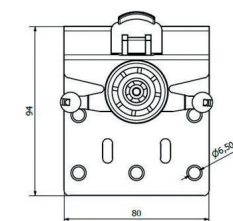
Top roller
