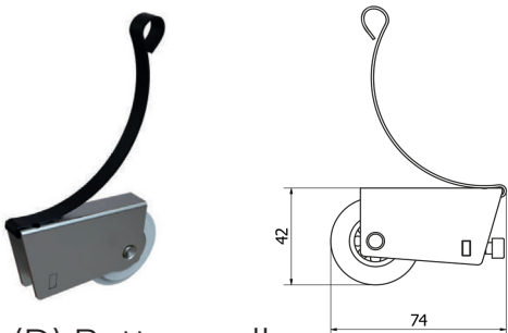
(D) Bottom roller Code: 500-202
